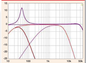
die Bandpassweichen und der Boost der 500.2 arbeiten sauber. Noch nicht perfekt ist das Tiefpassfilter der Class-D-Schaltung, das bei 50 kHz noch mal hochkommt. Das ist der Vorserie geschuldet und wird noch gefixt
