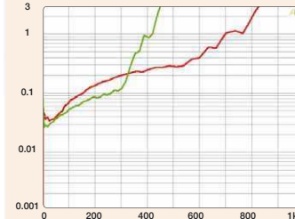
Auch als Bassendstufe nimmt die 750.1 ihren Job ernst: Es gibt sehr wenig Verzerrungen, dafür jede Menge Leistung bis 776 W an 2 Ohm
