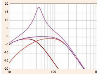
Die QL750.1-24V bietet mit Subsonic, Boost und Tiefpass alles, was geht
