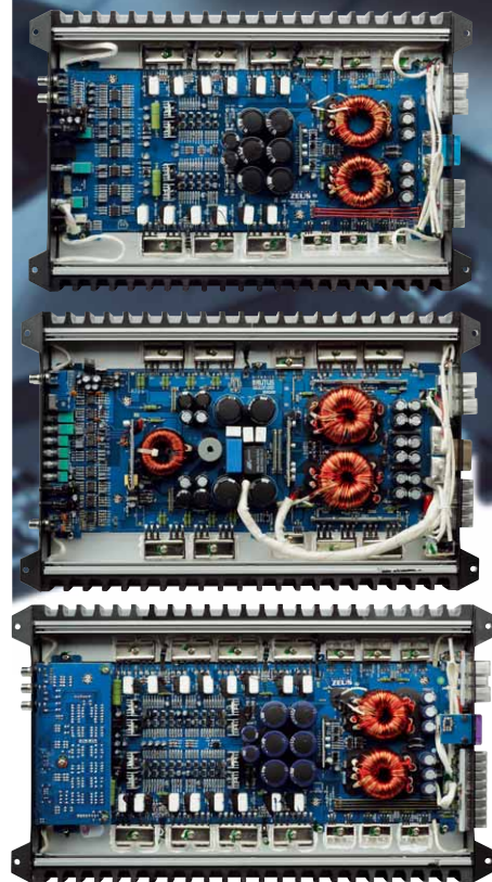
Die neuen Hifonics sind ganz klassisch aufgebaut mit sauberem Layout und guten Bauteilen. Die Brutus (mitte) verfügt über das kräftigste Netzteil
